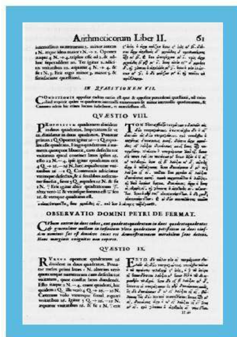
Problema 8 del libro II de la Arithmetica de Diofanto con comentarios de Fermat.
