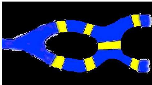
Puentes de Königsberg.
